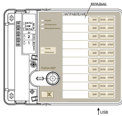
Рисунок 1 – Внешний вид и способ подключения прибора
